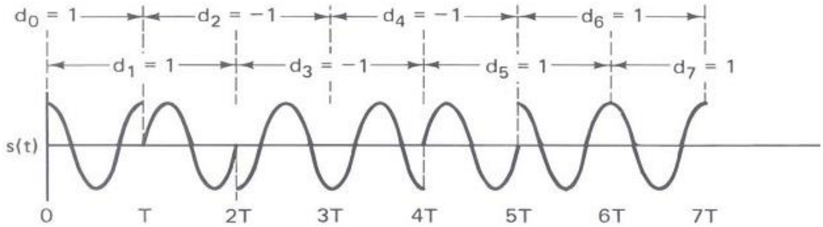
(b) OQPSK
